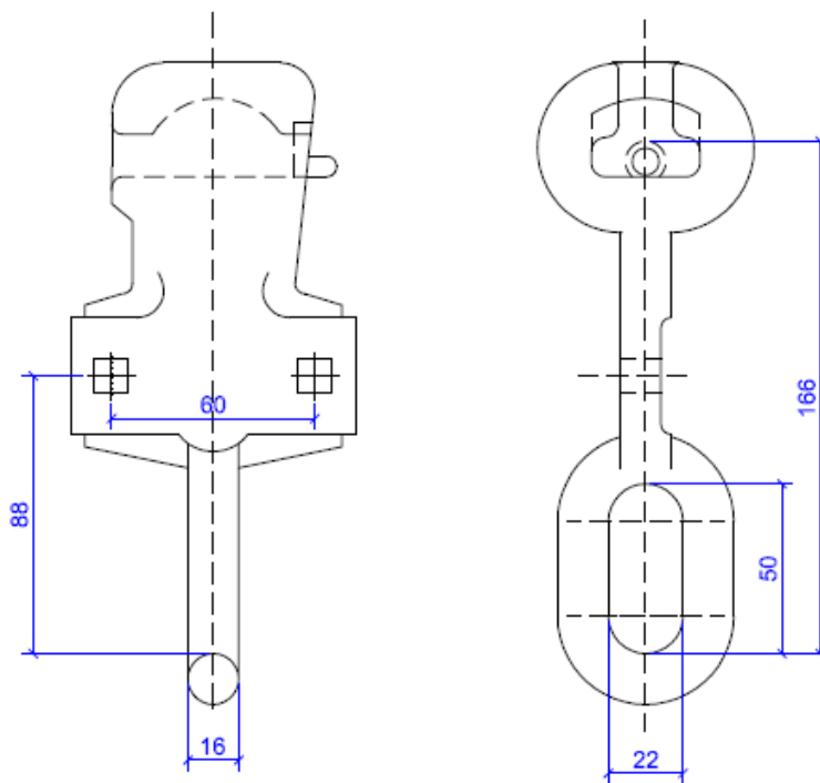
Figura 1 – Concha-Elo 90° com Suporte
